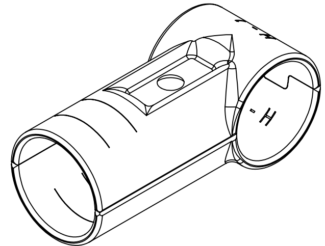
Isometrico
